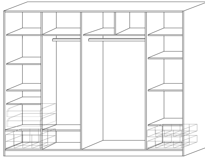
Šatník 2500 - příklad použití polic 500, dělicí svislé příčky, drátěných košů, zásuvek.
