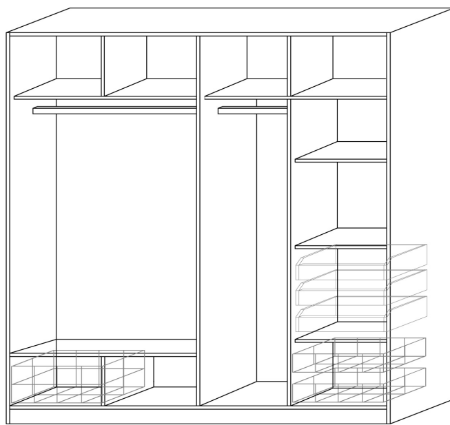
Šatník 2000 - příklad použití polic 500, dělicí svislé příčky, drátěných košů, zásuvek a zásuvkového modulu T.
